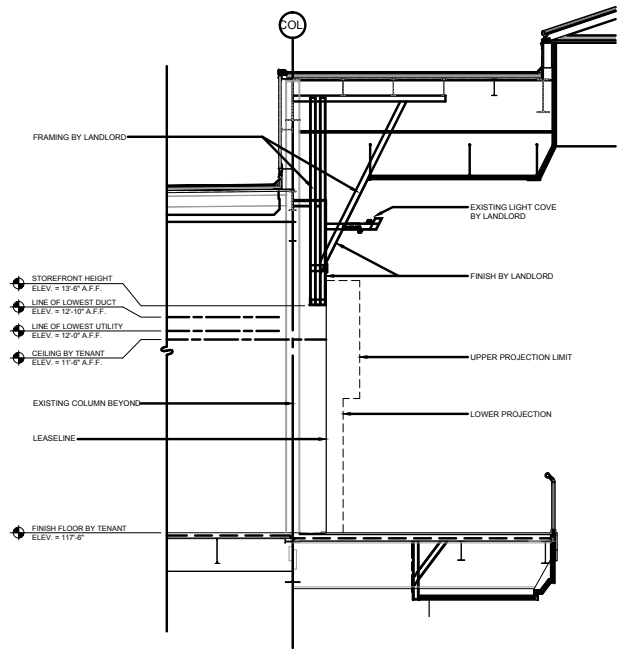
TYP. SECTION
