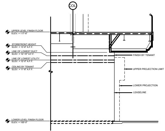
TYP. SECTION
