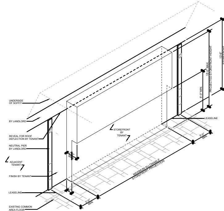
TYP. ISOMETRIC
