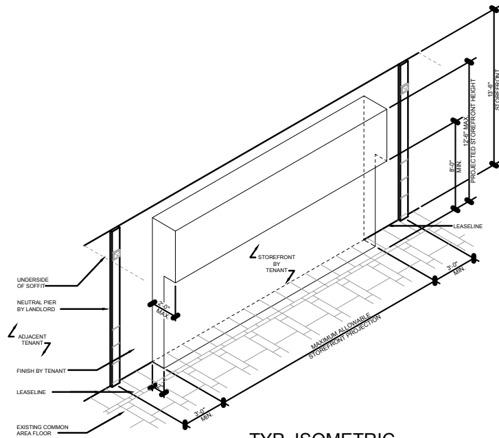
TYP. ISOMETRIC
